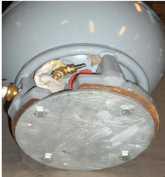
Bildet 1. Halon kule med tilkoblet plate.
